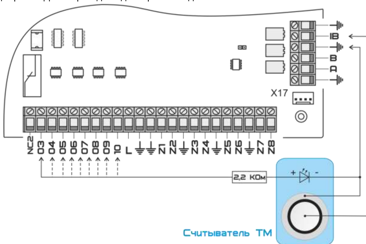
Рисунок 3.6. Схема подключения считывателя с одноцветным светодиодом.
