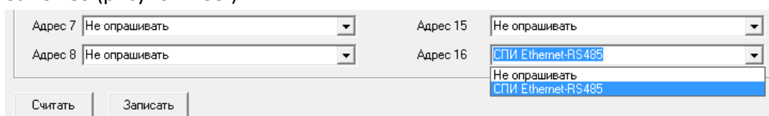
Рисунок 2.53. Подключение Ethernet модуля к ППКОП.
