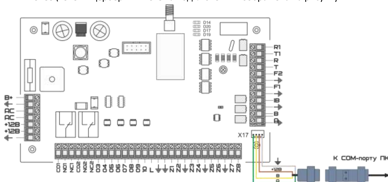
Рисунок 1.1. Схема подключения «Цербер» к ПК с использованием преобразователя интерфейса.
