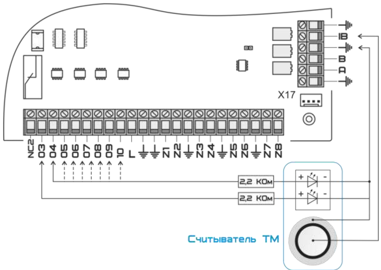
Рисунок 3.7. Схема подключения считывателя с двухцветным светодиодом.
