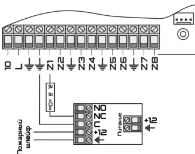
Рисунок 4.6. Схема подключения пожарных извещателей через M412NL.
