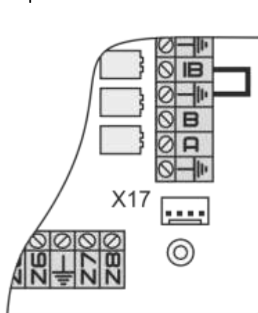
Рисунок 2. Установка перемычки для программирования параметров СПИ.
