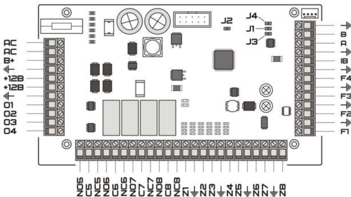
Рисунок 2.46. Схема выходов расширителя «Цербер Р».
