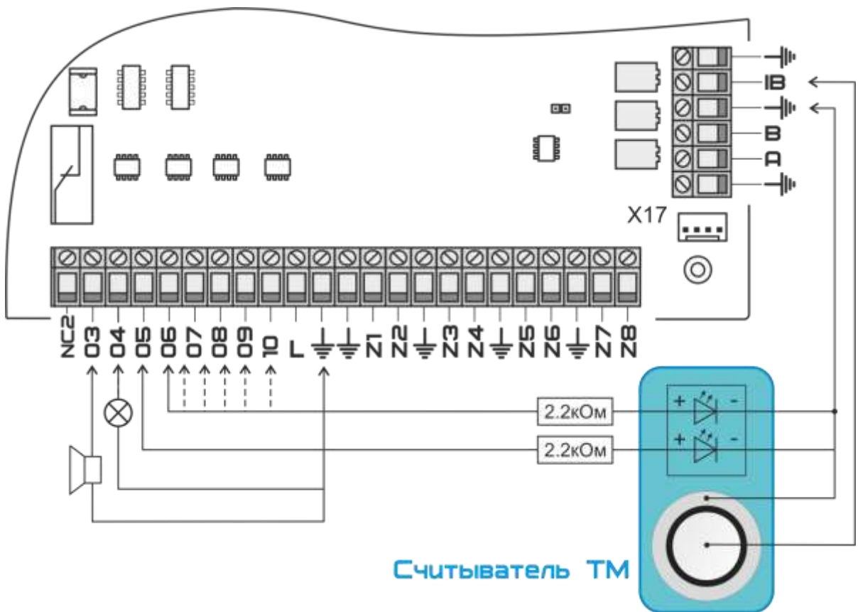
Рисунок 4.7. Схема подключения считывателя ТМ с 2-мя светодиодами и оповещателями.
