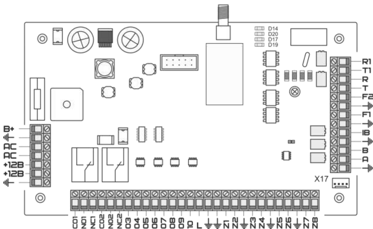
Рисунок 1.1. ППКОП «Цербер».
