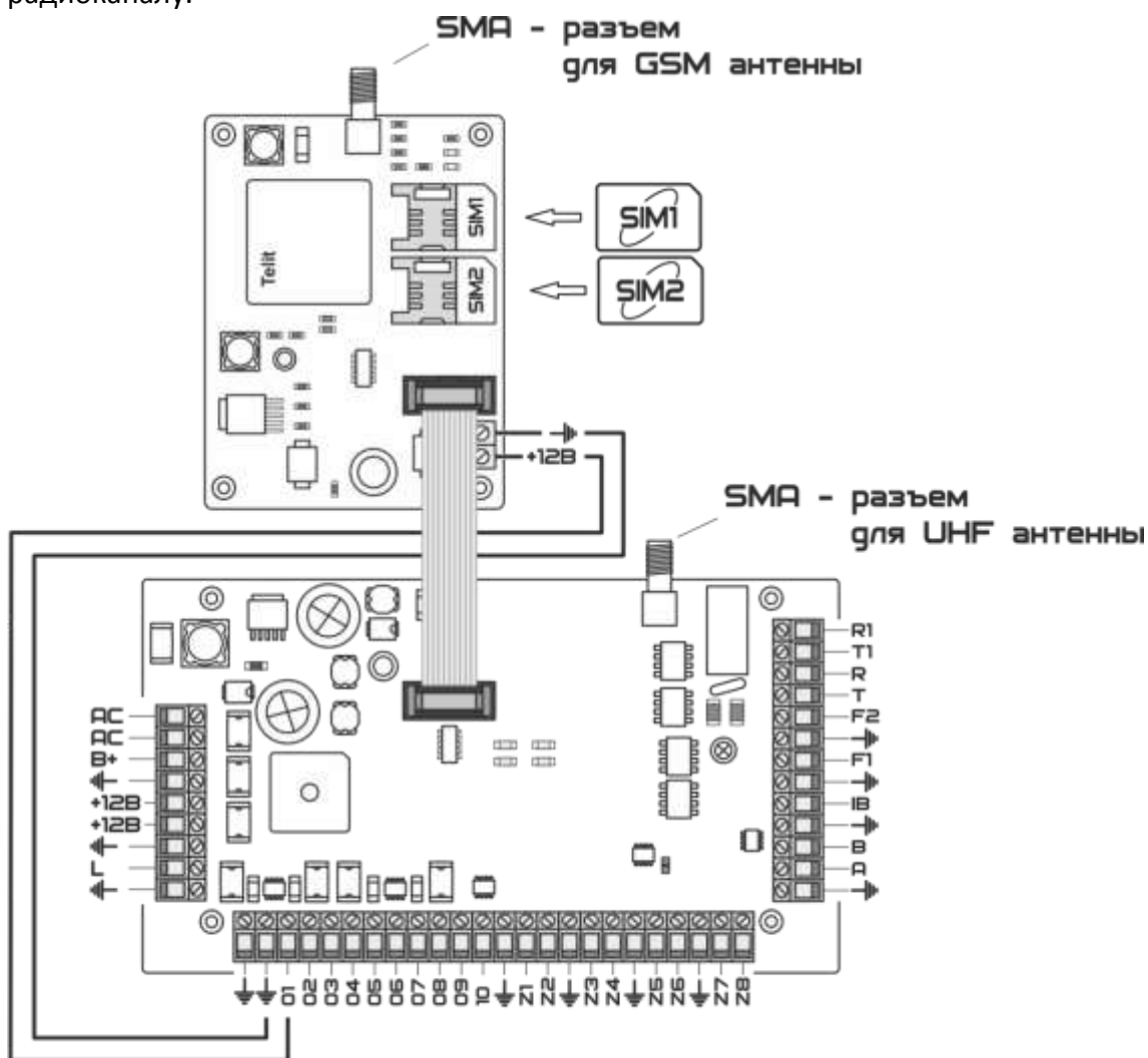
Рисунок 2.18. Схема подключения GSM модуля к ППКОП «Цербер».
